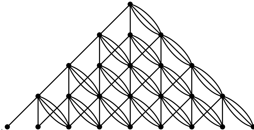
Рис. 1. Диаграмма Браттели, заданная производящим полиномом 1 + x + 3x^2 .
