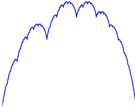
Рис. 2. Графики функции \mathcal{T}_{1/3}^1 .
